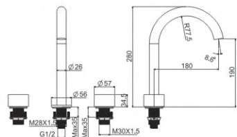
M82929LSJ Basin faucet
