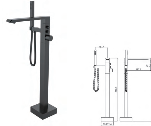
M93016-383H Freestand bath faucet
