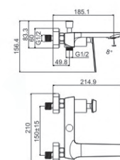
M31797-847LSJ Bath faucet
