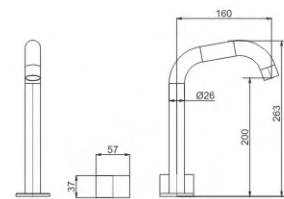
M81928LSJ Basin faucet
